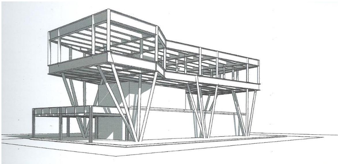
Perspectiva en Otra vista de la Propuesta Estructural, imagen de Tania Frausto Sandoval
