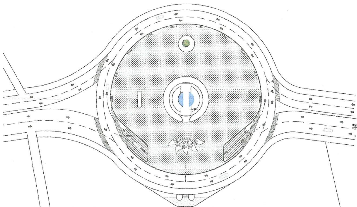
Planta general de Glorieta Arco de Bienvenida Imagen de Roberto Carrillo Chávez
