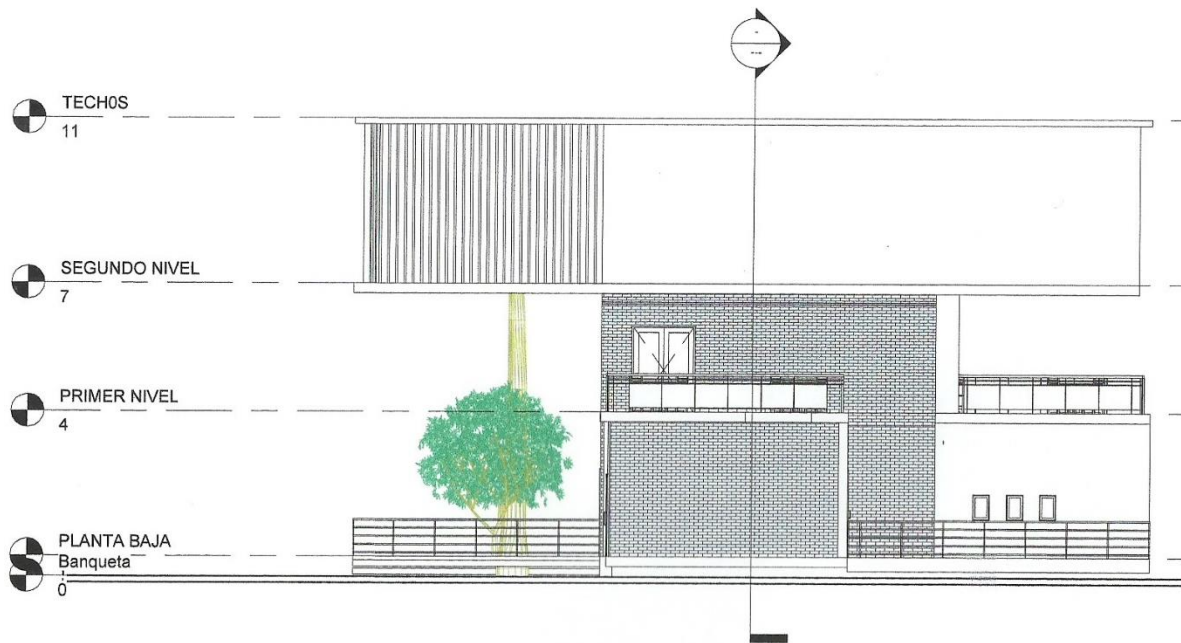
Fachada Este del Museo del Ferrocarril y Academia de Arte, imagen de Tania Frausto Sandoval
