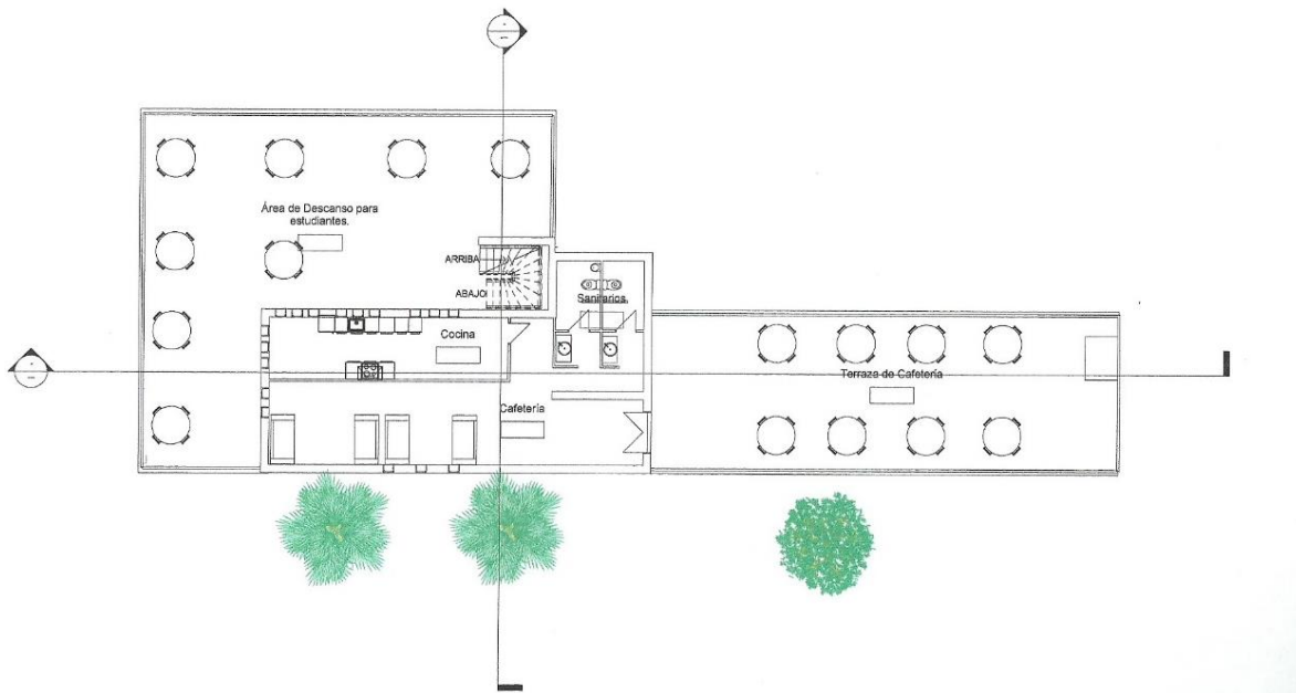
Plano de Primer Nivel del Museo del Ferrocarril y Academia de Arte, imagen de Tania Frausto Sandoval
