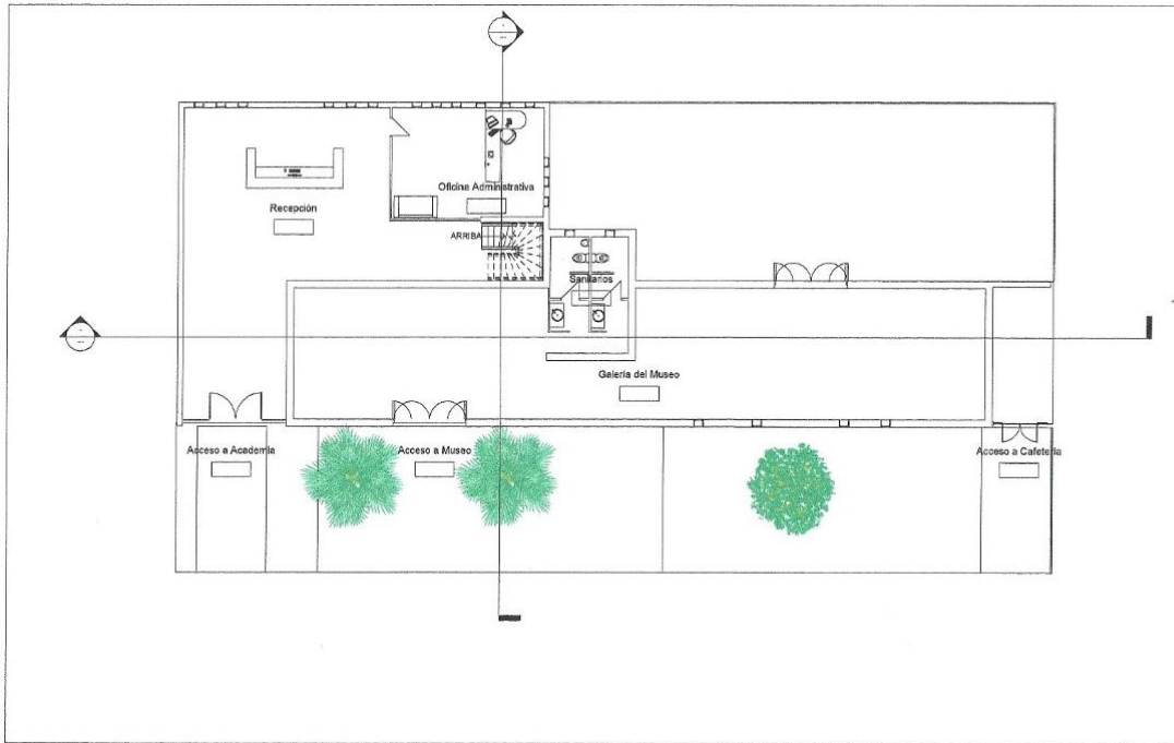
Plano de Planta Baja del Museo del Ferrocarril y Academia de Arte, imagen de Tania Frausto Sandoval
