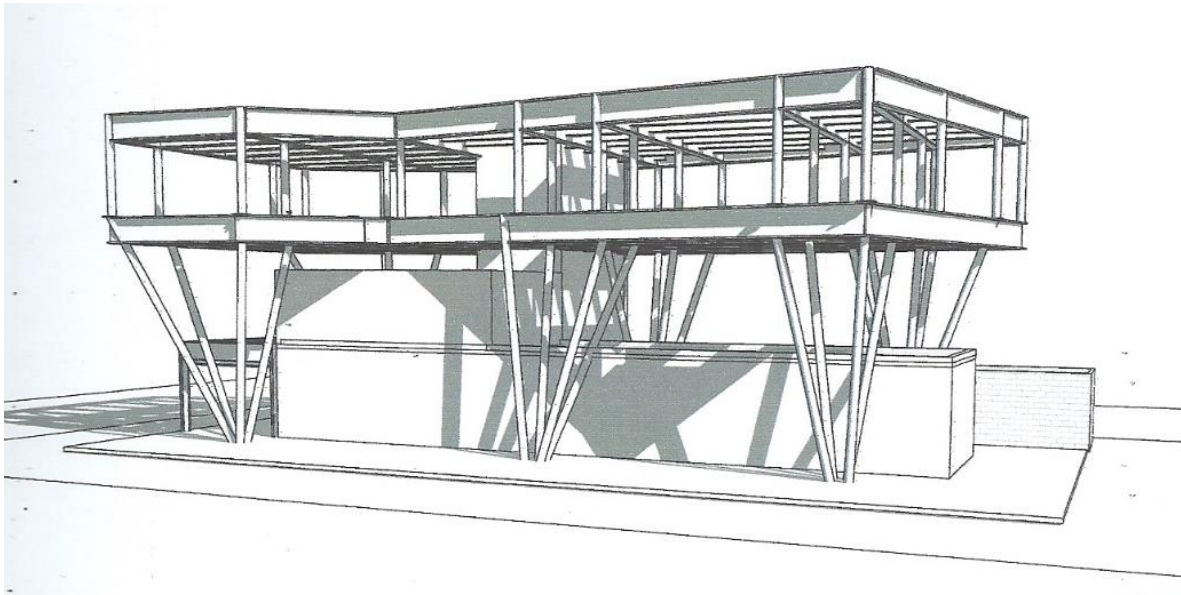
Perspectiva de la Propuesta Estructural, imagen de Tania Frausto Sandoval
