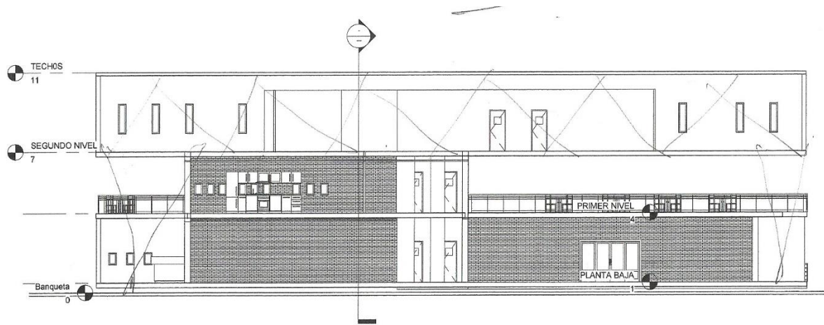
Corte Longitudinal del Museo del Ferrocarril y Academia de Arte, imagen de Tania Frausto Sandoval
