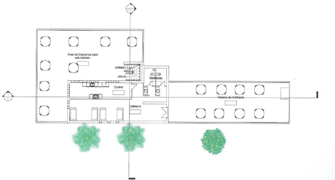
Plano de Primer Nivel del Museo del Ferrocarril y Academia de Arte, imagen de Tania Frausto Sandoval
