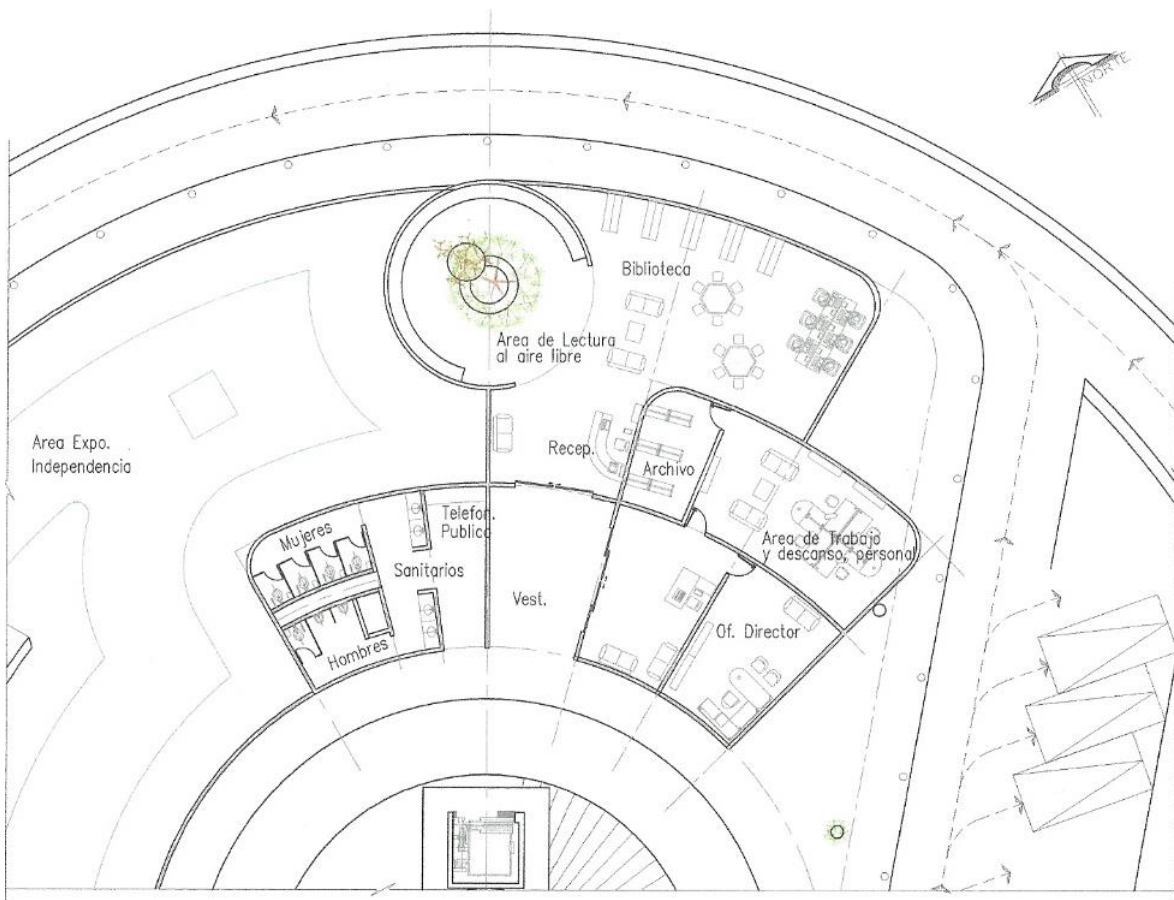
Detalle Área Administrativa, imagen de Roberto Carrillo Chávez
