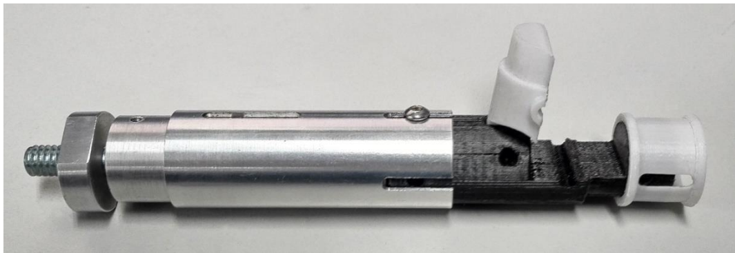
Foto 2. Perno de ABS (Acrílico Butadieno Estireno) por impresión en 3D. constituido por tres piezas: el cuerpo, la mordaza y el seguro
